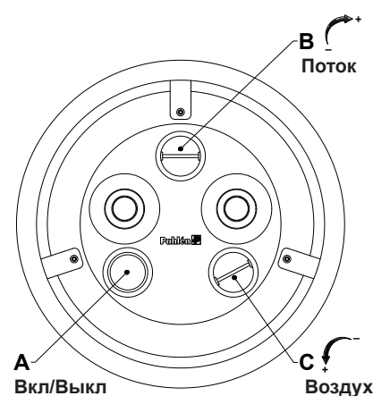
Рис.1. Перед.панель Jet Swim 2000
